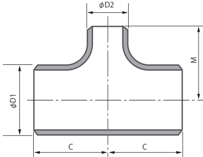
径違いT
