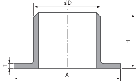
ラップジョイント
