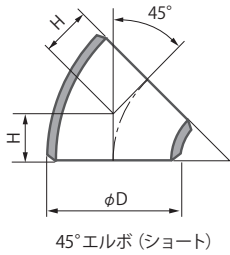
45°エルボ (ショート)
