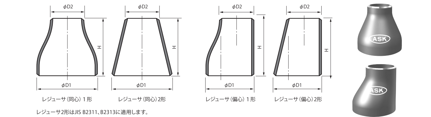
レジューサ2形はJIS B2311、B2313に適用します。
