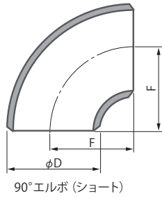
90°エルボ (ショート)
