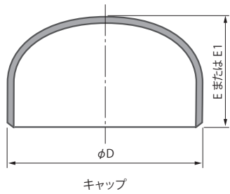
キャップ
